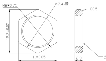
Nut
