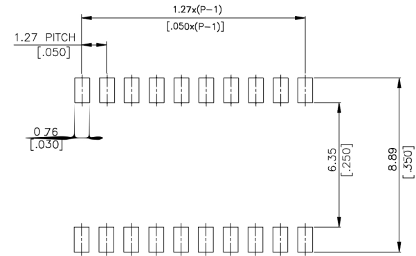
P.C.B. LAYOUT
