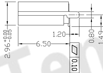
加胶帽示意图
