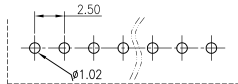
P.C.Board Layout
